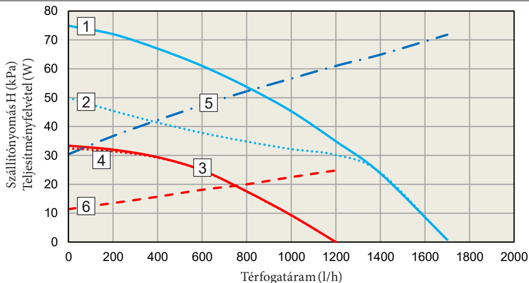
Grafikon Térfogatóram - Emelőmagasság - Teljesítményfelvétel Victrix Tera V3 38 EU
