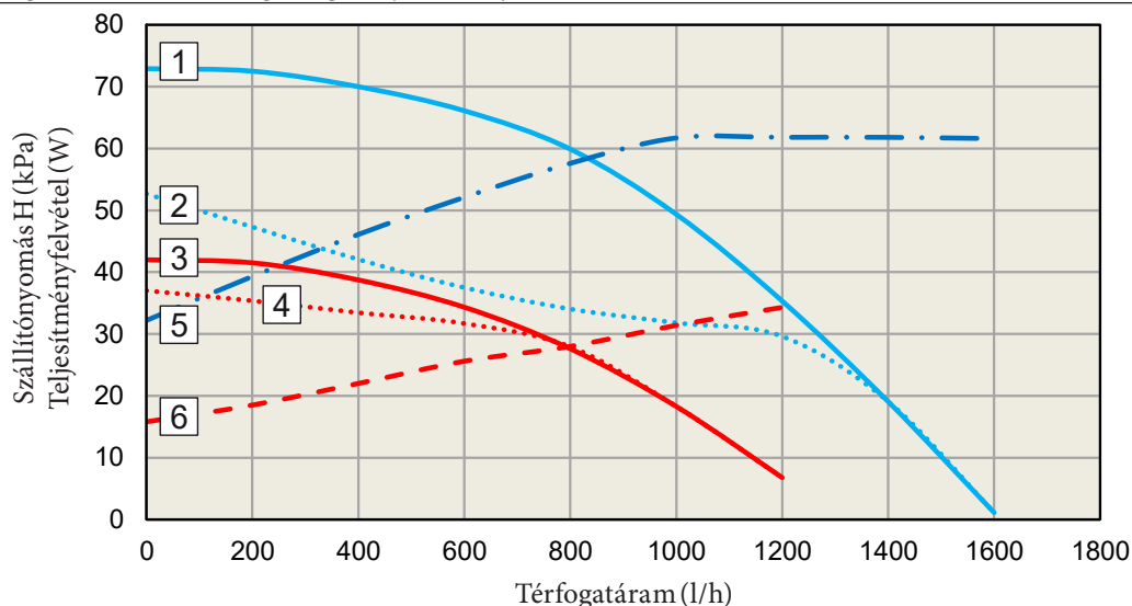
Grafikon Térfogatóram - Emelőmagasság - Teljesítményfelvétel Victrix Tera V3 32 EU
