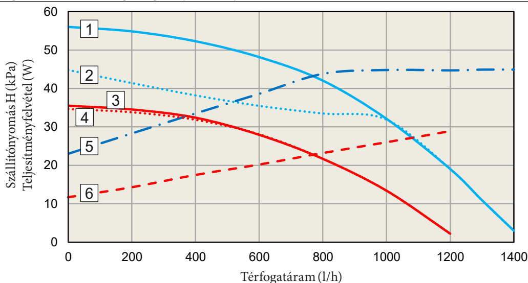
Grafikon Térfogatáram - Emelőmagasság - Teljesítményfelvétel Victrix Tera V3 28 EU
