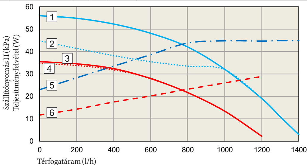
Grafikon Térfogatáram - Emelőmagasság - Teljesítményfelvétel Victrix Tera V3 24 Plus EU
