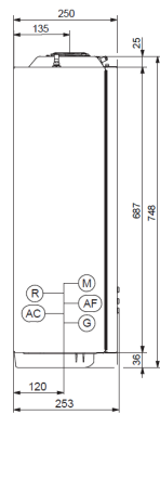
VICTRIX TERA V3 28 / 32 csatlakozási méretek
