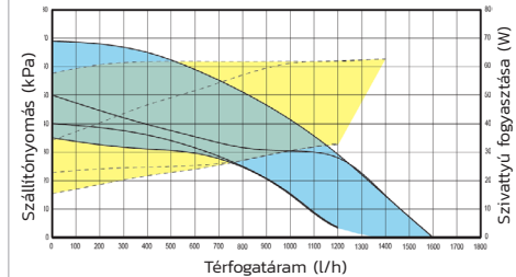
VICTRIX TERA V3 32 és 35 Plus szivattyú jelleggörbe
