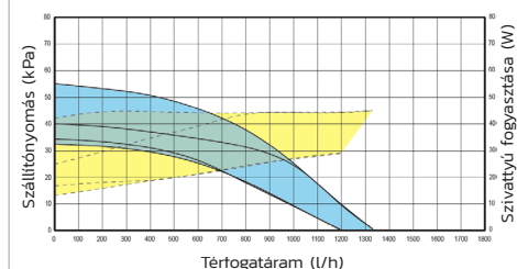
VICTRIX TERA V3 32 és 35 Plus szivattyú jelleggörbe
