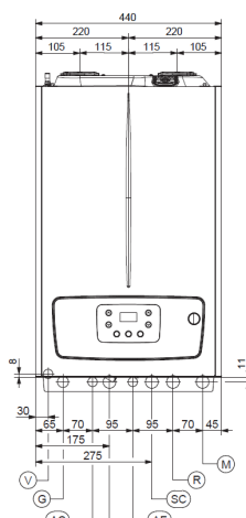
VICTRIX TERA V3 28 / 32 csatlakozási méretek
