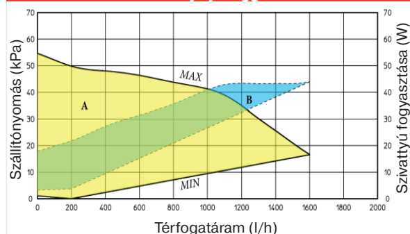
Szivattyú jelleggörbe
