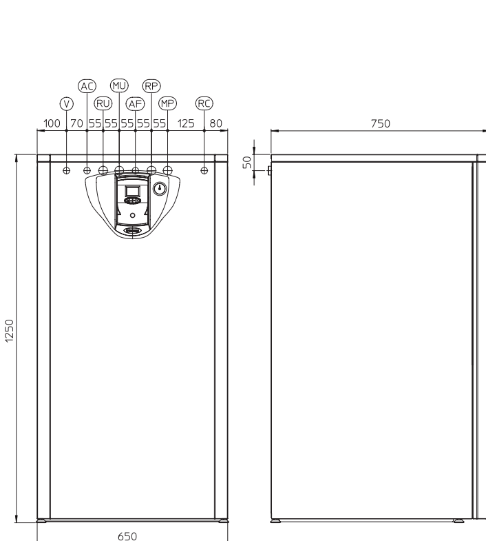
UB 200 Solar indirekt HMV tároló méretei
