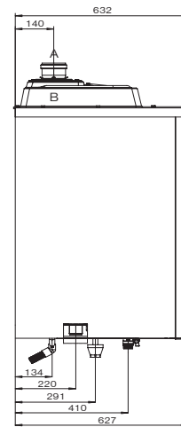
VICTRIX PRO 100 és 120 ErP
