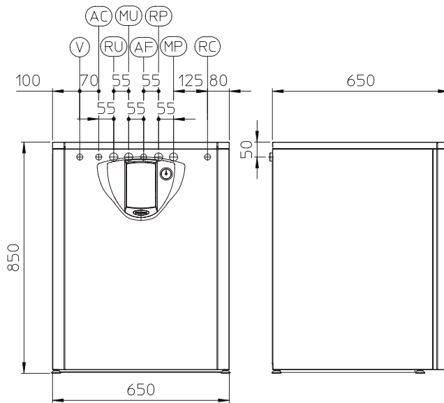
UB 120 indirekt HMV tároló méretei
